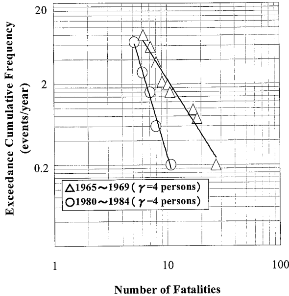
Fig. 4 Modified risk curve considering a location parameter of \gamma for boiler accidents. 位置パラメータを入れたリスク曲線 (ボイラー災害)
