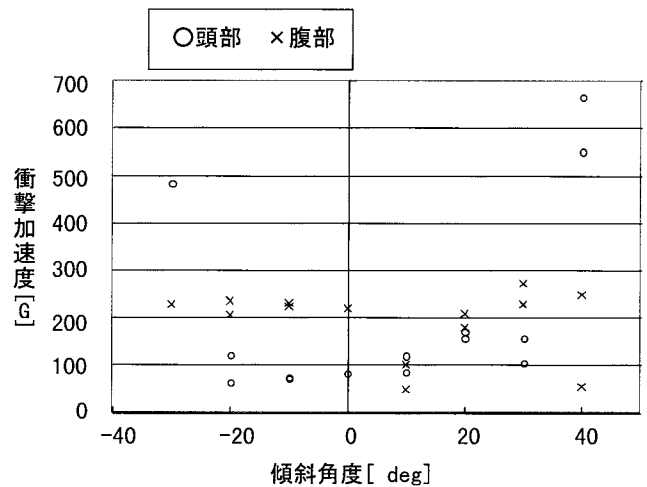
Fig. 9 Shock and fall posture. 落下姿勢や衝撃加速度
