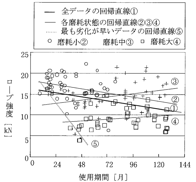
Fig. 2 Duration of service and strength of lanyard. 使用期間とランヤード強度
