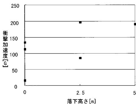
Fig. 12 Shock in standing posture. 立位落下時の衝撃加速度
