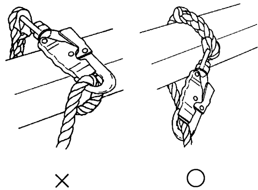
Fig. 5 Usage of hook (2) 回し掛けの方法
