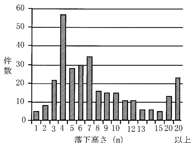
Fig. 7 Number of fall accident on fall height basis. 落下高さごとの墜落件数
