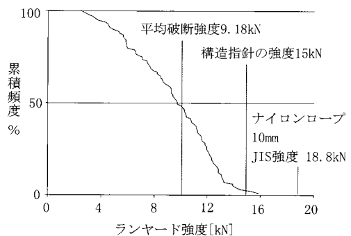
Fig. 1 Strength of lanyard of used safety belts. 使用した安全帯のランヤードの強度
