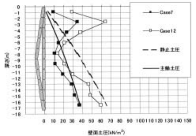
Fig. 33 Distribution of lateral earth pressures on wall. 壁面土圧の分布状況（ X/L=0.040 ：中央）
