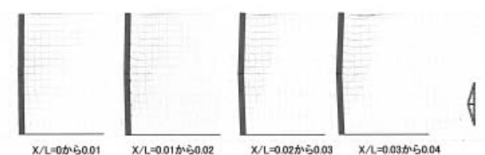
Fig. 7 Visualized deformation area in Case3 (crank mode). 変位領域の可視化画像 (Case3)
