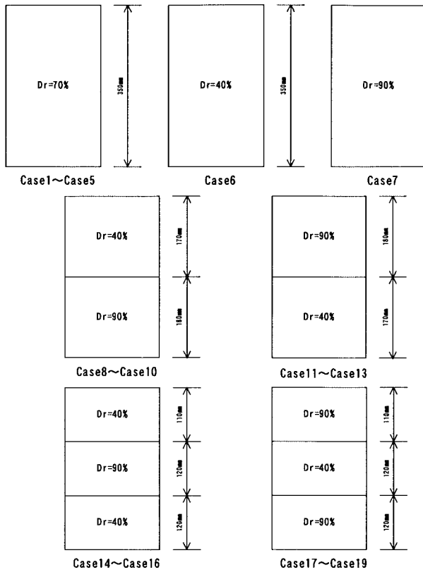
Fig. 3 Stratum conditions for each model. 模型地盤層毎の地盤条件
