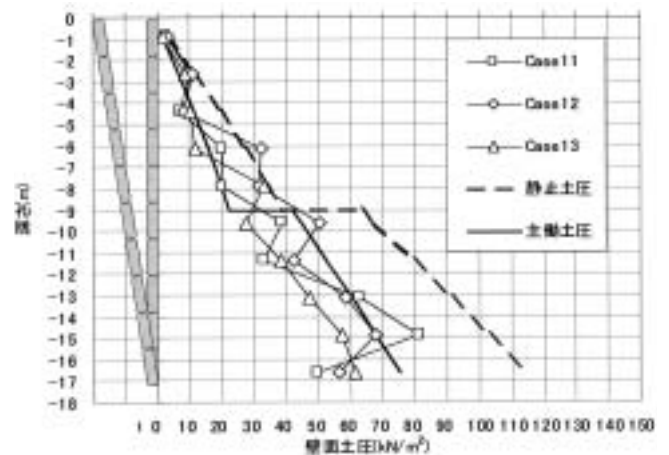
Fig. 34 Distribution of lateral earth pressures on wall. 壁面土圧の分布状況（ X/L=0.040 ：中央）
