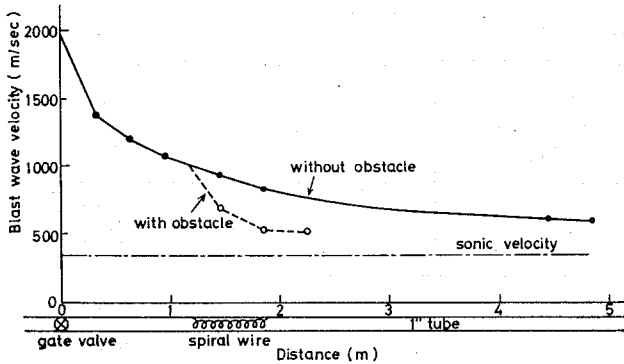
Fig. 8 Effect of spiral obstacle on blast wave propagation in air in 1 inch tube. The blast wave was driven by equimolar oxy-acetylene detonation. 衝撃波伝播速度に及ぼす管路の障害物の影響、アセチレン-酸素等モル混合ガスの爆ごう波を1インチ管中空気へ打ち込んだ場合
