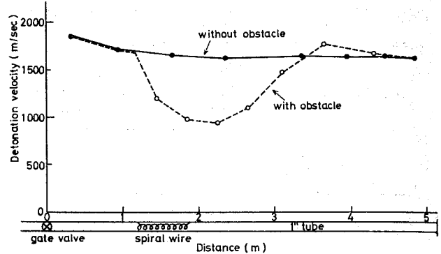
Fig. 9 Effect of spiral obstacle on detonation propagation of H 2 20% in air in 1 inch tube. The detonation was driven by equimolar oxy-acetylene detonation. 爆ごう伝播速度に及ぼす管路の障害物の影響、アセチレン-酸素等モル混合ガス爆ごう波で1インチ管中のH 2 20%-空気混合ガスを起爆した場合
