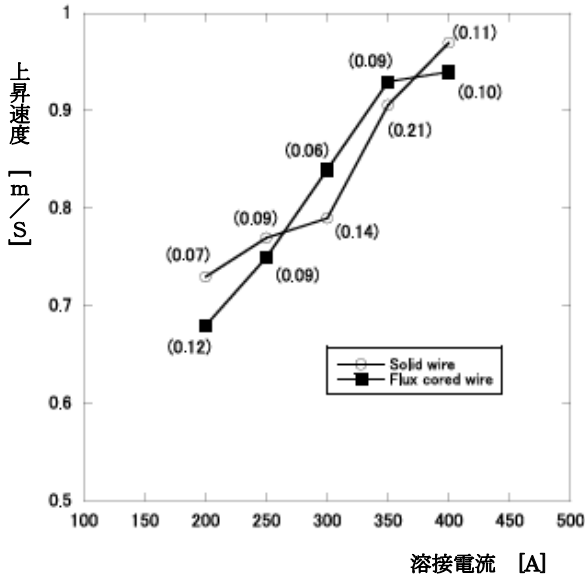
図1 ヒューム上昇速度と溶接電流の関係
