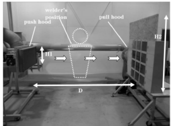
図2 開放型プッシュプル型換気装置の配置例
