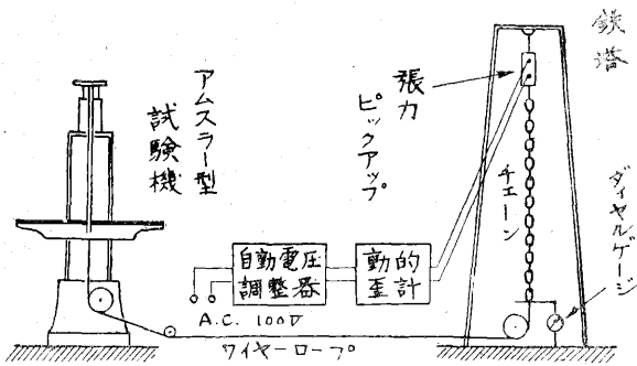
第2図 衝撃系の伸び測定装置
