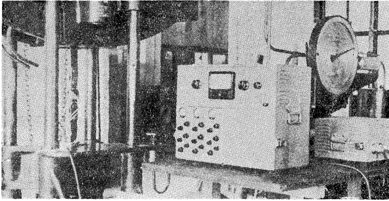
第1図 張力ピックアップの較正
