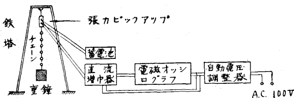
第3図 衝撃荷重測定装置
