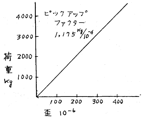
第 3 図 ピックアップの特性
