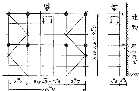
第1図 実験足場規模図
