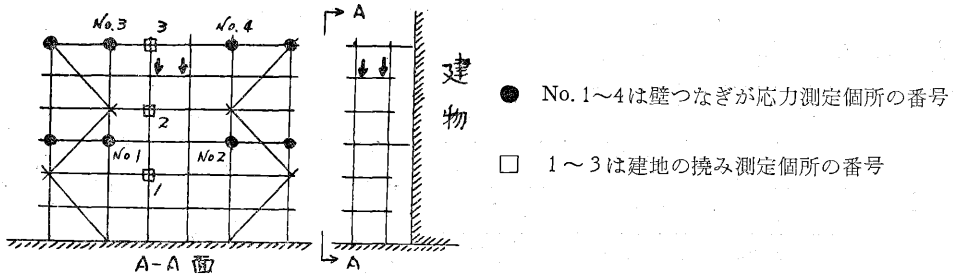
第 2 表 (1) 壁つなぎを上下二段に設けた場合
