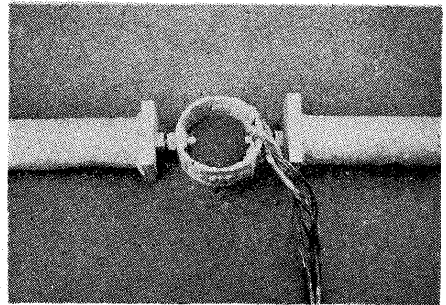
写真 3 プルービングリング
