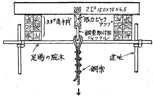
第 4 図 張力ピックアップ取付図
