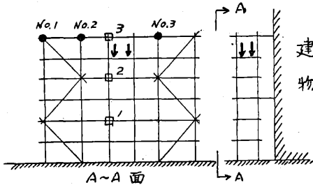
第3表 (2) 壁つなぎを上段のみに設けた場合
