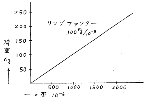
第 5 図 プルービングリング No. 2 の特性
