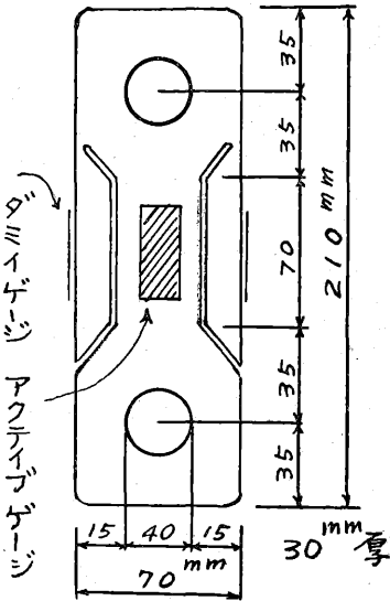
第 2 図 歪計ゲージを貼り付けた張力
