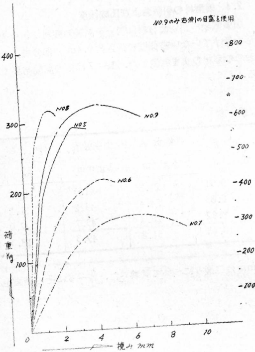
図-18 レール荷重-撓み線図
