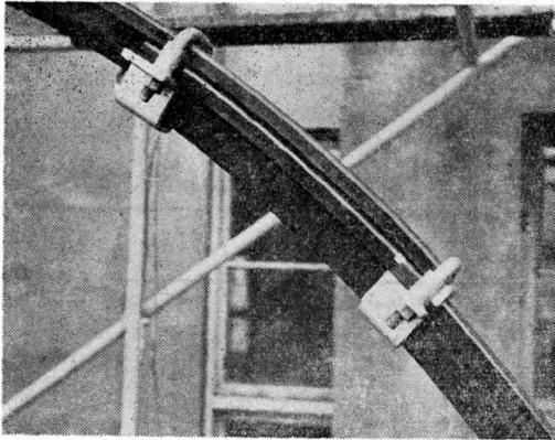
図-3 可溶接手
