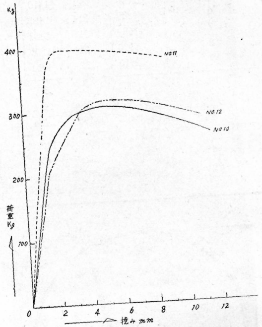
図-19 V形鋼の荷重-撓み線図
