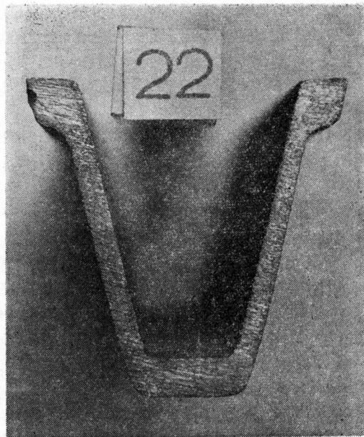
図-15 背高V形断面
