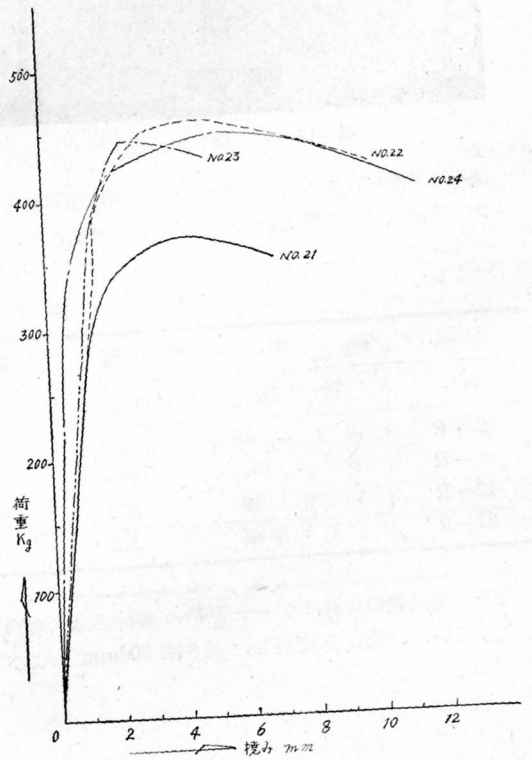
図-20 背高V形鋼の荷重-撓み線図
