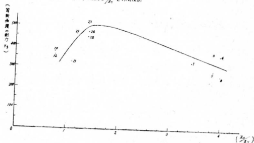
図-22 アーチの耐力と Z_x/Z_y との関係図
