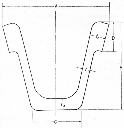
図-1 V形鋼断面
