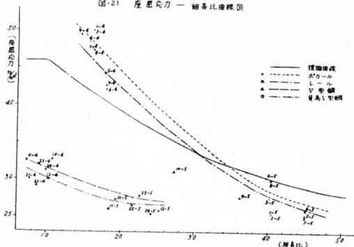
図-21 座屈応力-細長比曲線図
