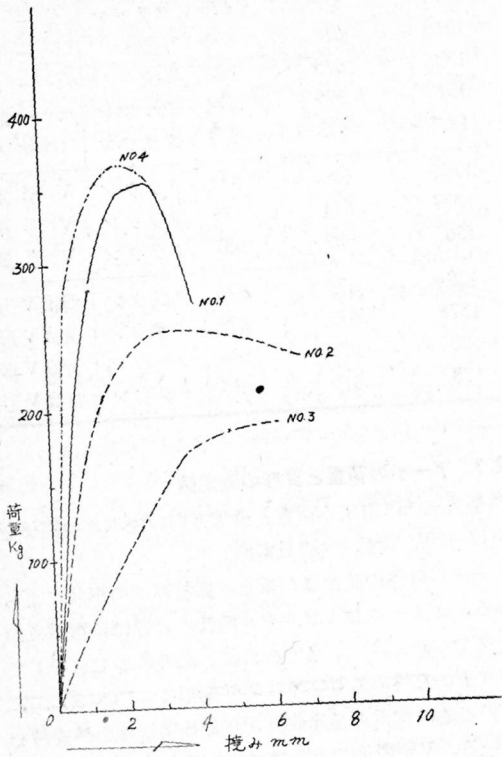
図-17 ポカールの荷重-撓み線図
