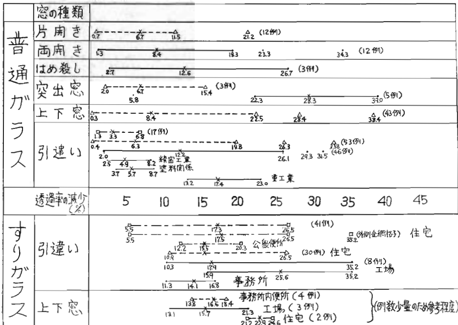
図2 種類別窓ガラス透過率測定
