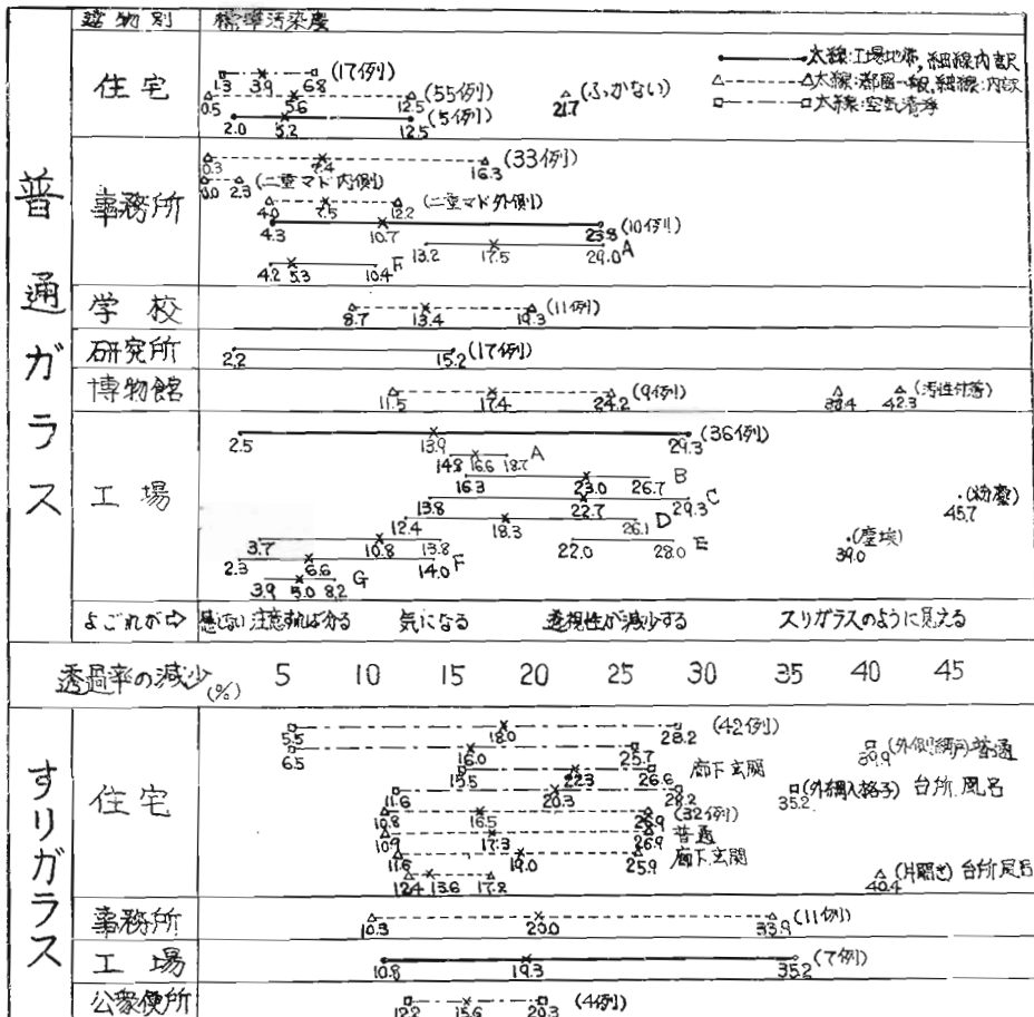
図3 建物別窓ガラス透過率測定
