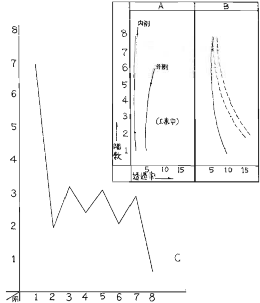
図4 窓の階高による透過率の減少調査事例
