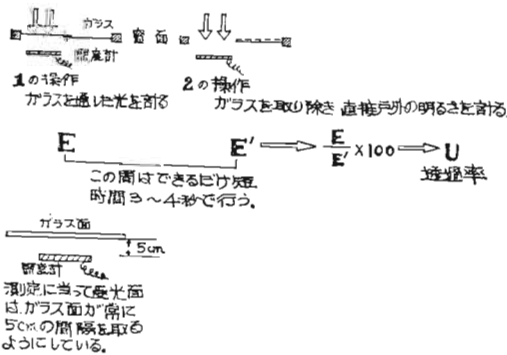
図1 光の透過率の測定模型図
